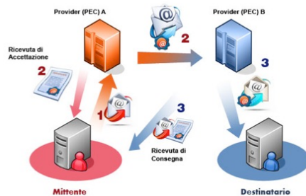
Fig 1. flusso PEC
